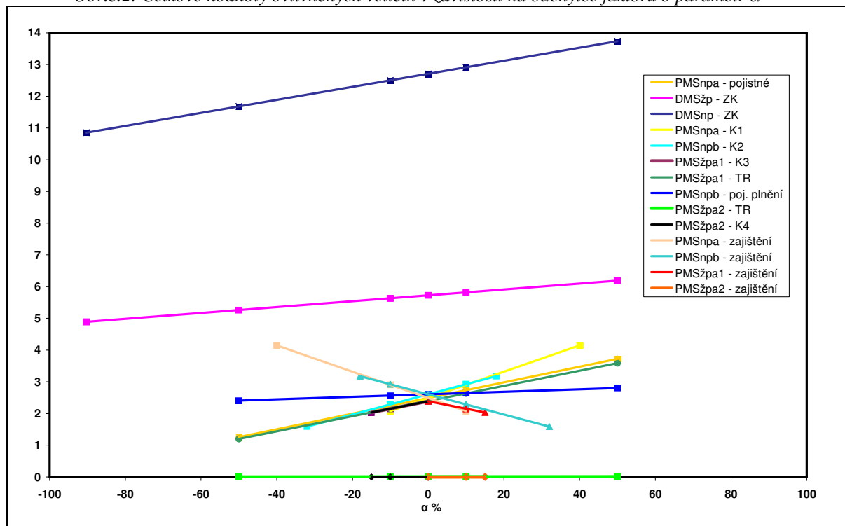
Obr.č.2: Celkové hodnoty ovlivněných veličin v závislosti na odchylce faktoru o parametru \alpha
