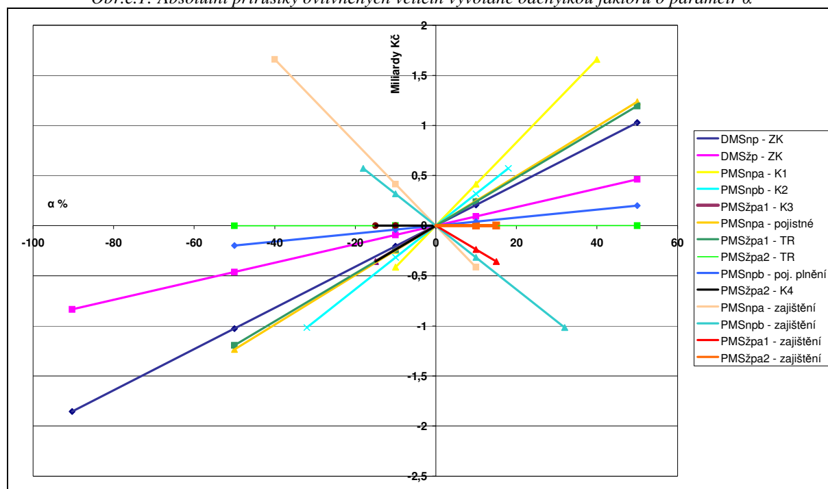
Obr.č.1: Absolutní přírůstky ovlivněných veličin vyvolané odchylkou faktoru o parametr \alpha
