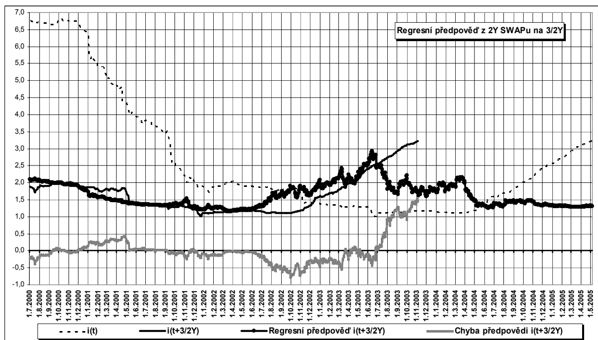
Obrázek č. 3: Předpověď 3M LIBORu na jeden a půl roku dopředu z hodnot 2Y SWAPu. Čárkovaná je skutečná neposunutá sazba 3M LIBOR, černě (tenká čára) tato sazba posunutá o 1,5 roku. Černá (silná čára) je předpověď podle výrazu (5), šedá čára kolem nuly je chyba této předpovědi.
